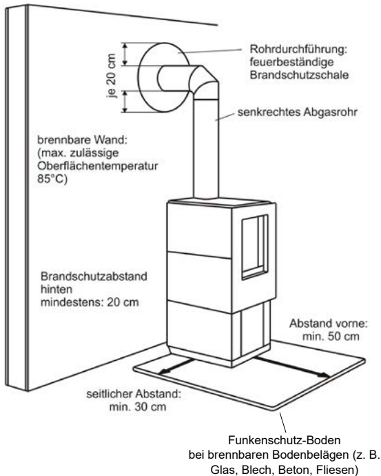
Sicherheitsabstände bei der Aufstellung von Kaminöfen im Wohnraum mit brennbaren Wänden und brennbaren Fußböden.
